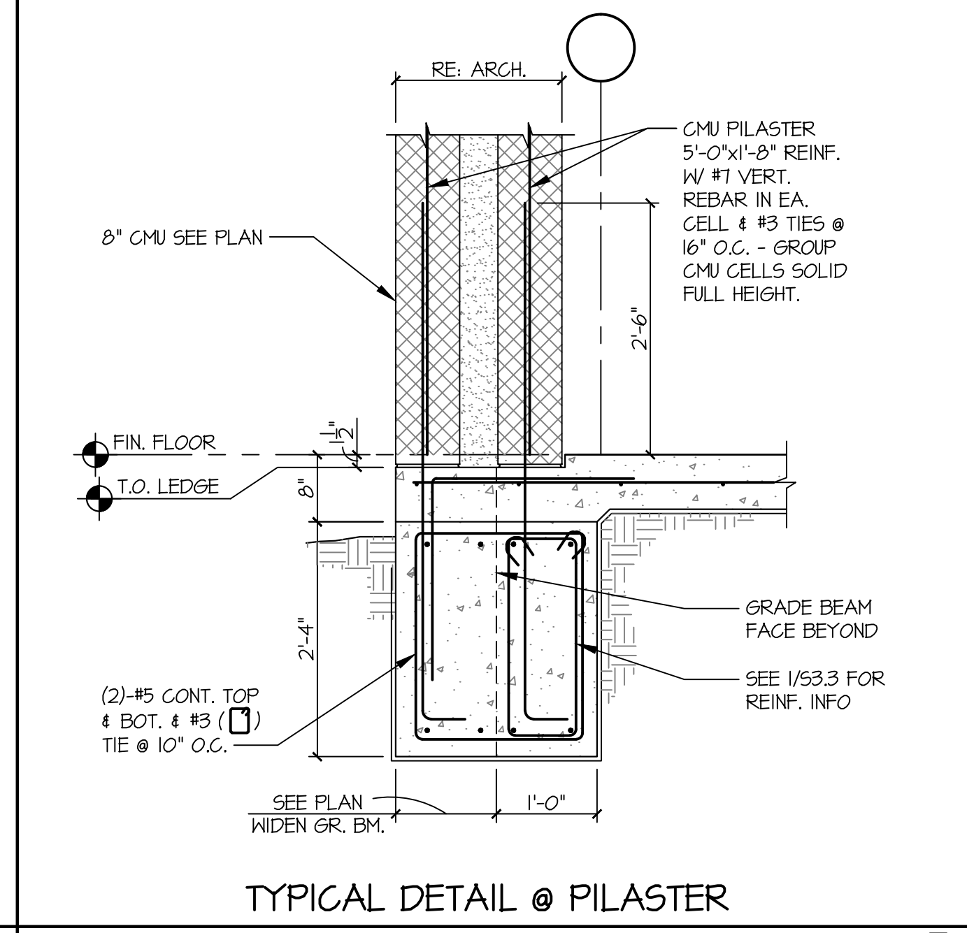
SCALE: 3/4" = 1'-0" 5
