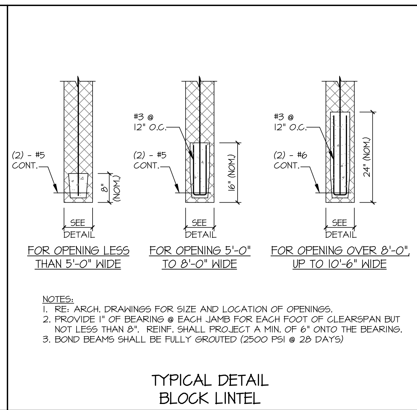
SCALE: 3/4" = 1'-0" 6
