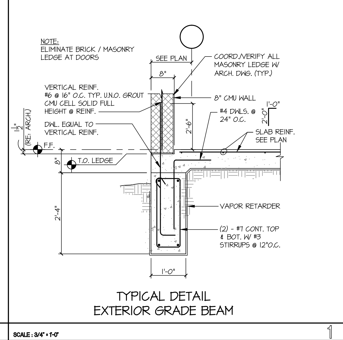
SCALE: 3/4" = 1'-0" 1
