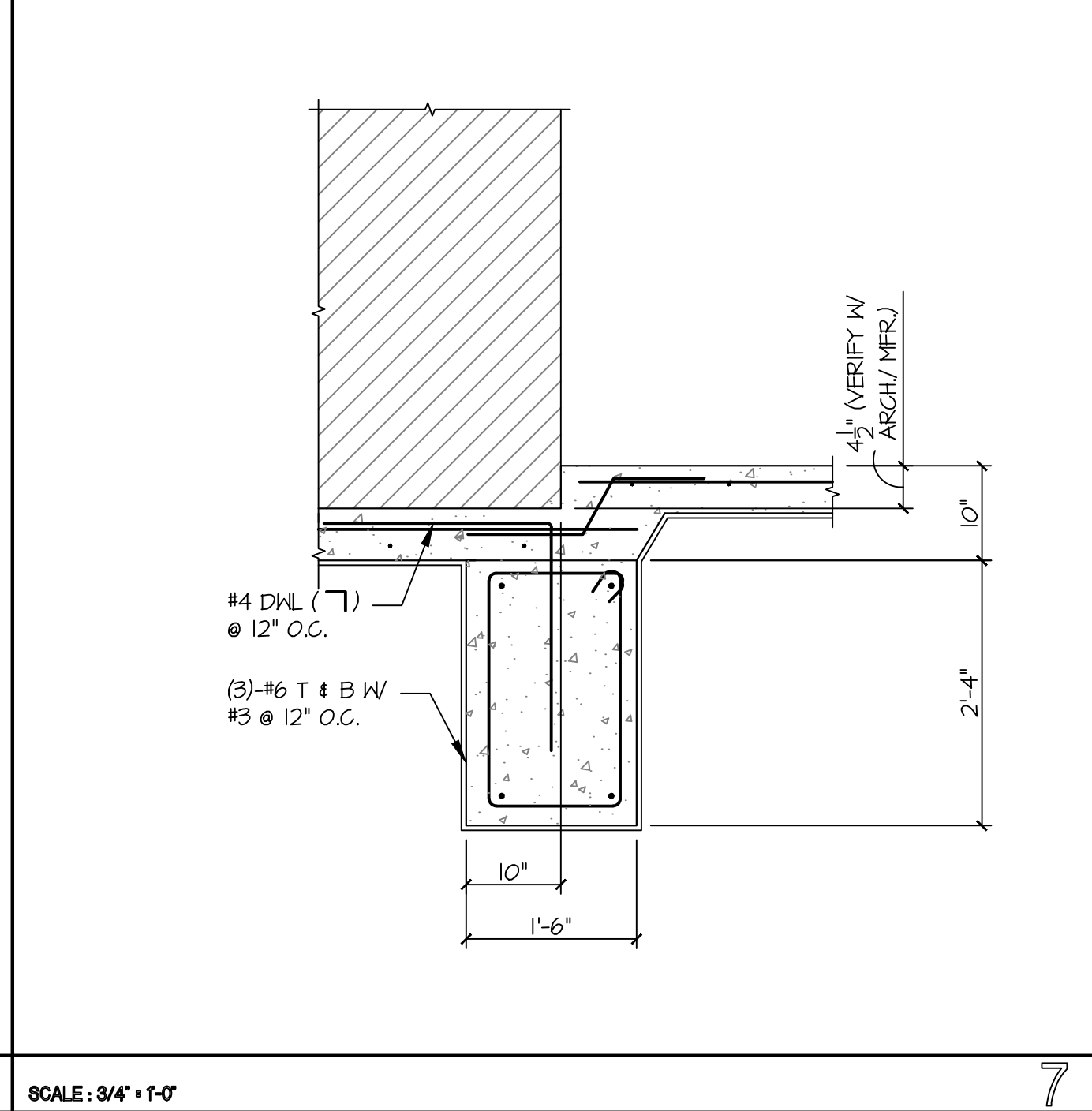
SCALE: 3/4" = 1'-0" 7
