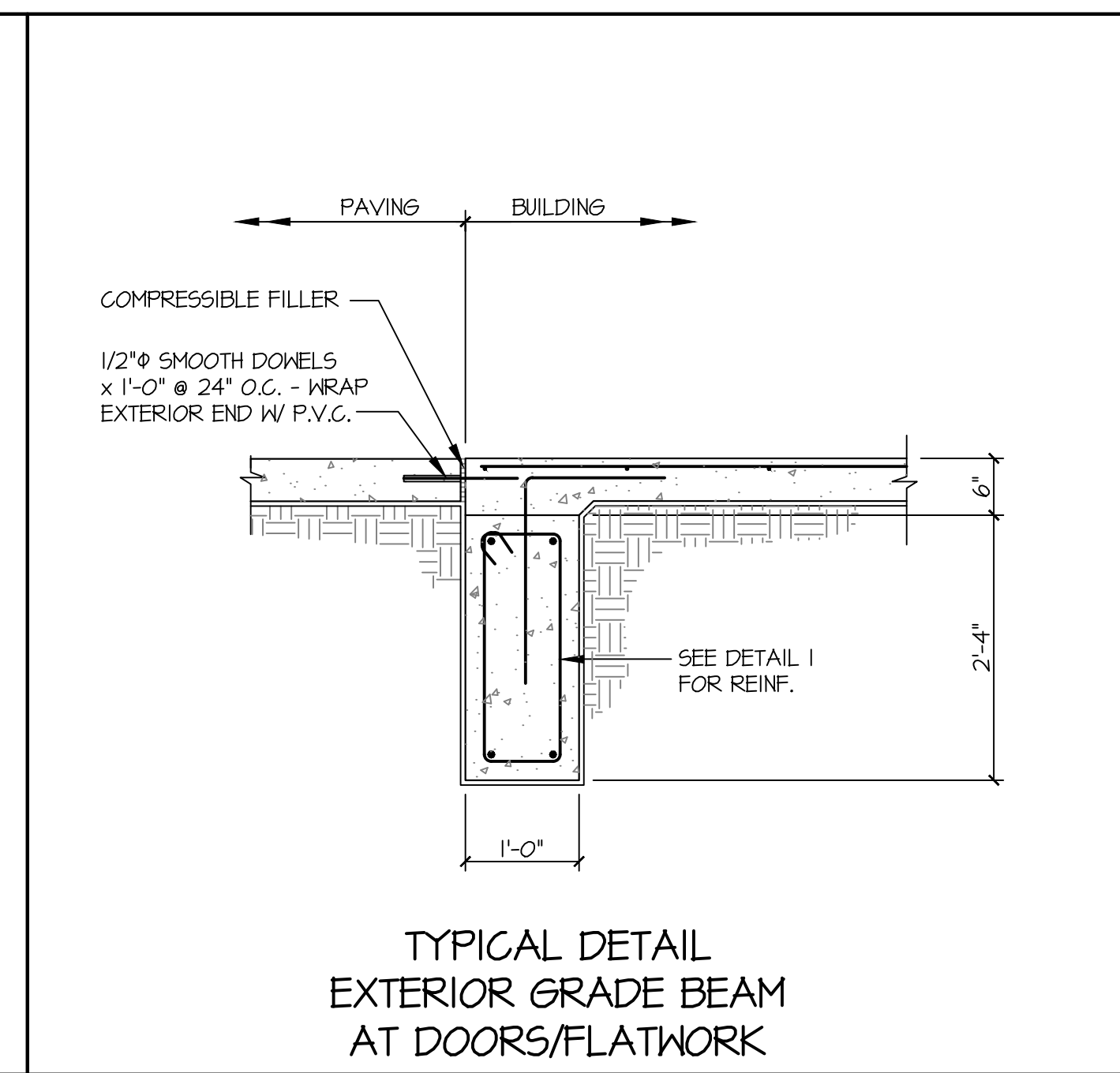
SCALE: 3/4" = 1'-0" 3
