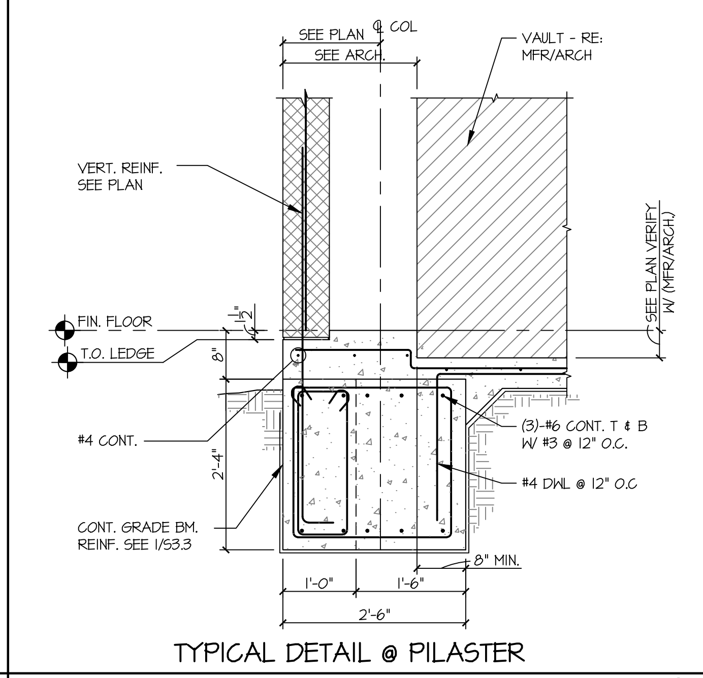
SCALE: 3/4" = 1'-0" 8
