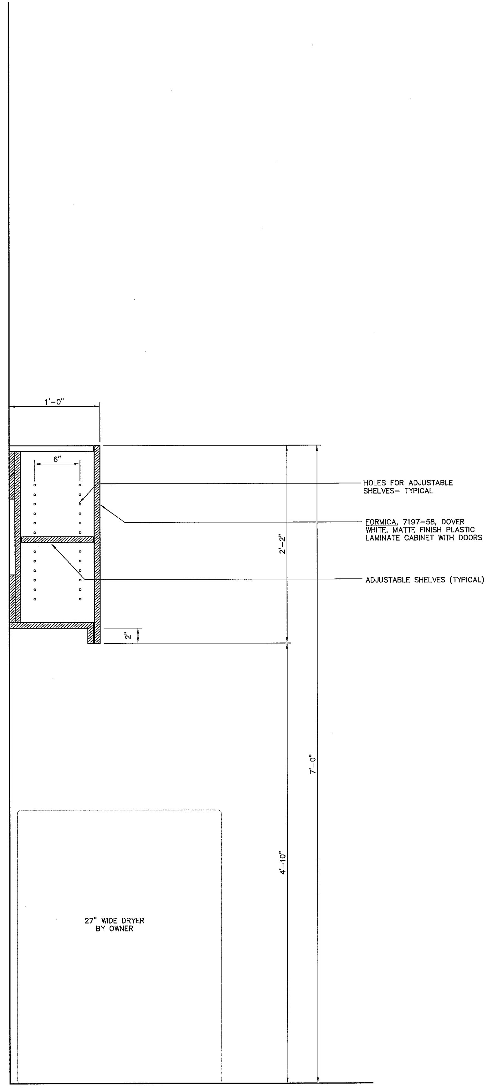
MILLWORK SECTION 02 SCALE: 1-1/2"=1'-0"
